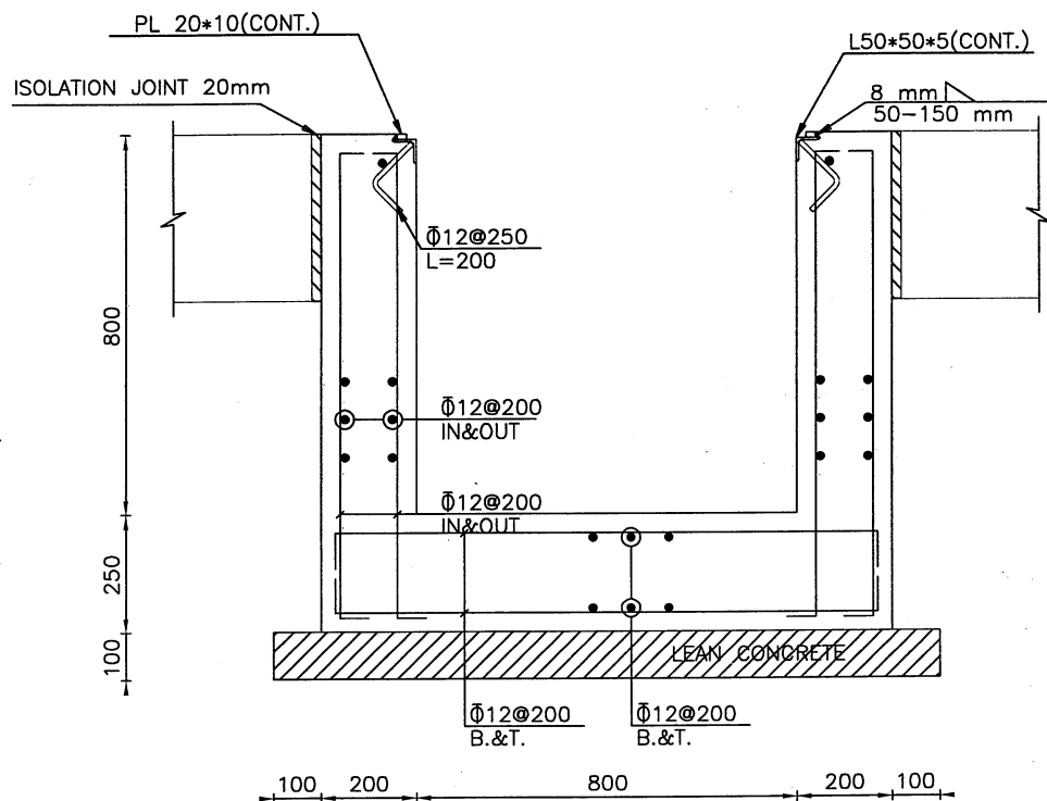
SECTION D-D
